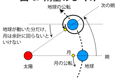
図 2: 朔望周期
